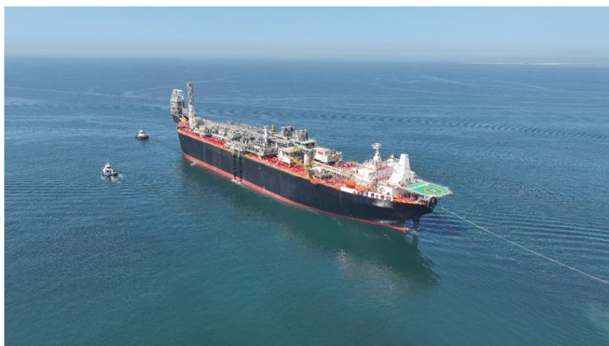
FPSO Baobab Ivoirien
